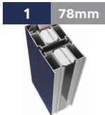
1 78mm Ciepła ościeżnica z poliamidową przekładką termoizolacyjną
